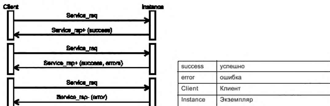
Рисунок 65 — Диаграмма последовательностей
