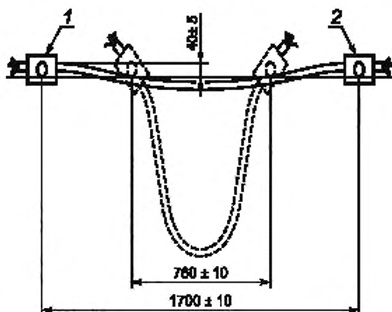
1 — зажим для кабеля; 2 — ось вращения зажима
