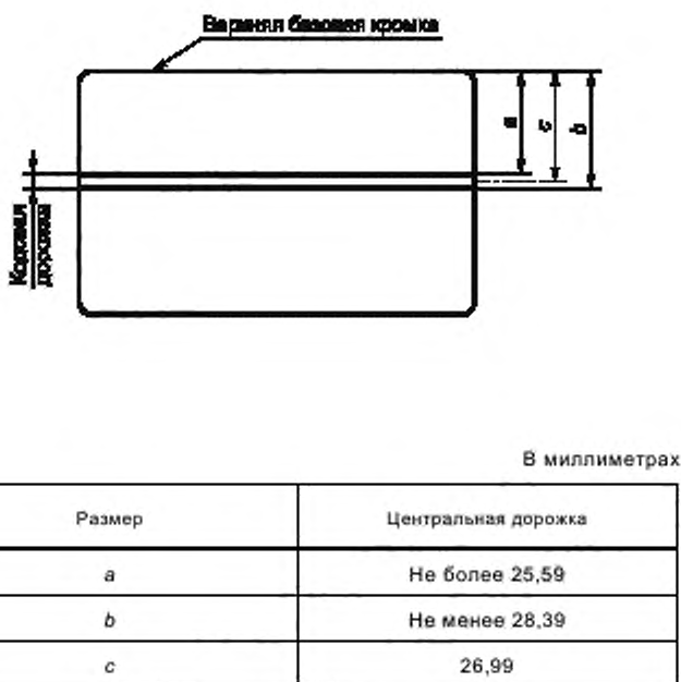
Рисунок 5 — Расположение центральной дорожки для карт форматом TFC.1
