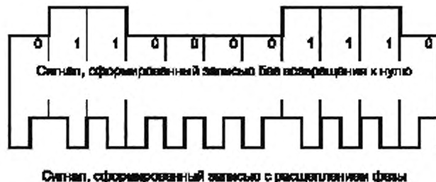
Рисунок В.2 — Кодирование с расщеплением фазы
