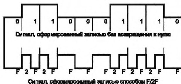
Рисунок В.1 — Кодирование F/2F
