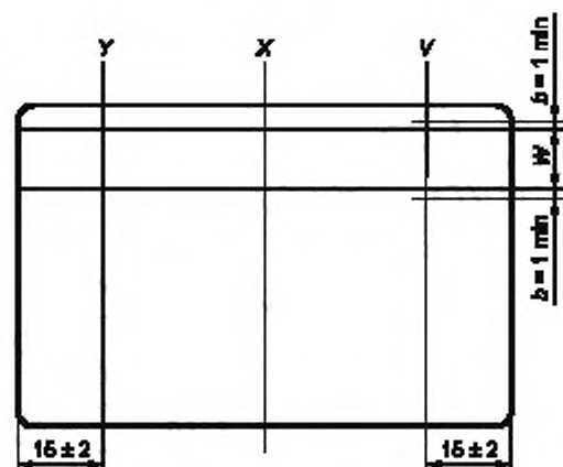
Рисунок 5 — Положение линий измерений профиля магнитной полосы
