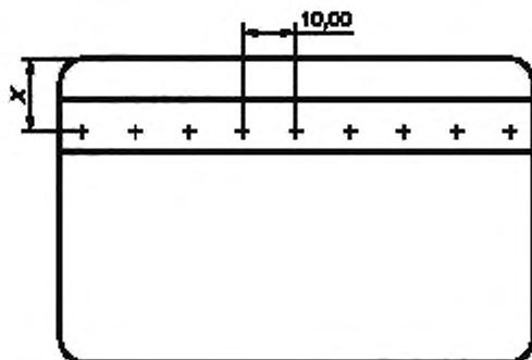
Рисунок 2 — Точки измерений
