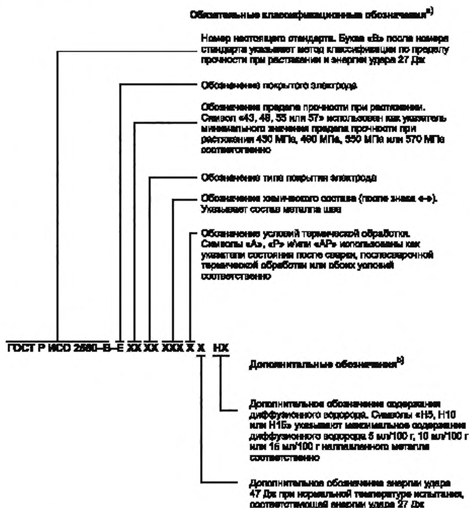
Рисунок А.2 — Обозначение электродов по ГОСТ Р ИСО 2560-В (классификация по пределу прочности при растяжении и энергии удара 27 Дж)
