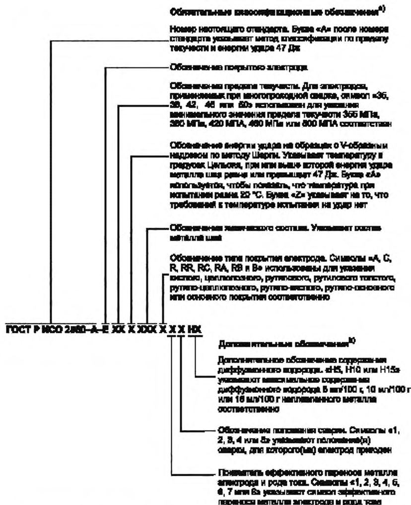
Рисунок A.1 — Обозначение электродов по ГОСТ Р ИСО 2560-A (классификация по пределу текучести и энергии удара 47 Дж)
