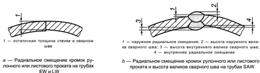
Рисунок 4 — Отклонения размеров сварного шва
