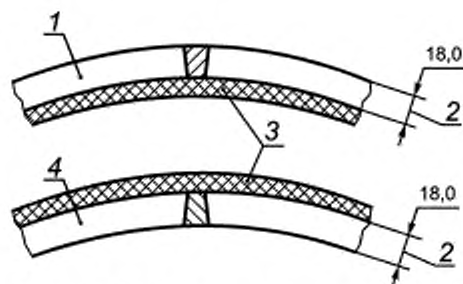
1 — загнутый образец с внешней стороны шва; 2 — уменьшенная толщина стенки; 3 — металл, удаляемый до или после выпрямления; 4 — загнутый образец с корнем шва
