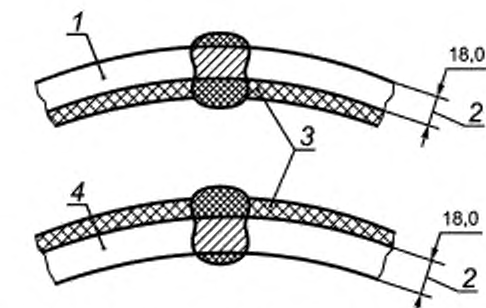
с — Образцы уменьшенной толщины стенки (по выбору, для труб SAW и COW толщиной стенки t > 19,0 мм)
