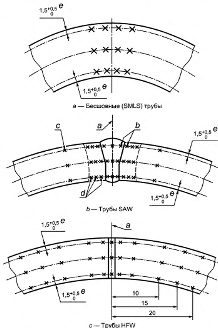
Рисунок J.1— Участки контроля твердости
