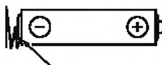
Рисунок В.10а — Пружина прокалывает отрицательную оболочку — возможен контакт с металлом
