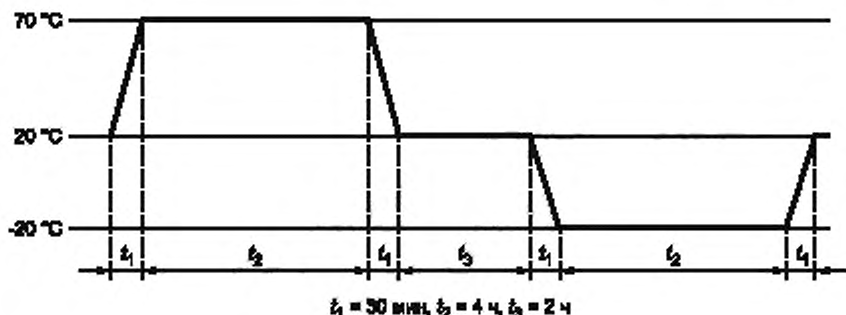
Рисунок 2 — Температурный цикл
