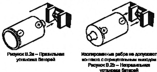
Рисунок В.2 — Положительный контакт, утопленный между ребрами
