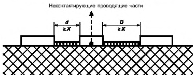
Рисунок E.7 — Несплошной стык с узкой и широкой канавками
