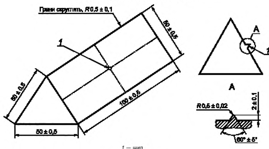
Рисунок 14 — Оправка
