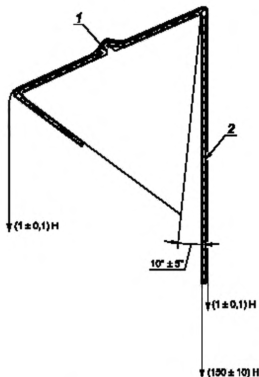
1 — шип; 2 — металлическая фольга
