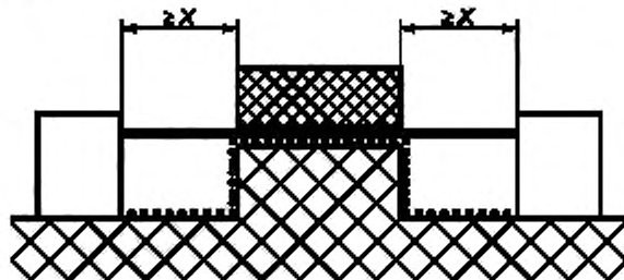
Рисунок E.5 — Неплотный стык с узкими канавками
