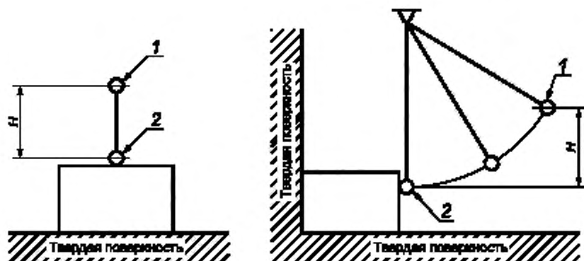
Рисунок 8 — Испытание на удар с использованием стального шара
