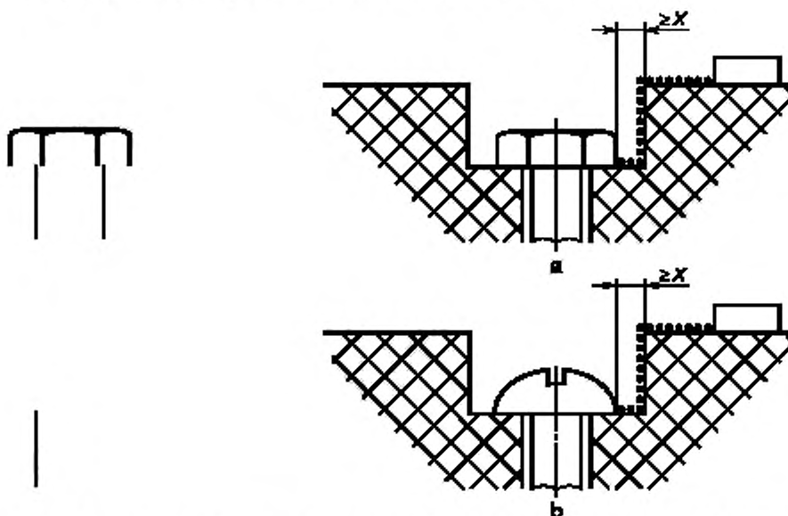
Рисунок E.8 — Промежуточная, несоединенная проводящая часть
