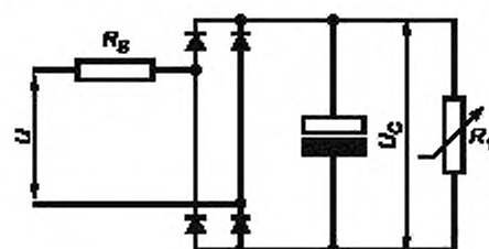
Рисунок М.4 — Эталонная нелинейная нагрузка
