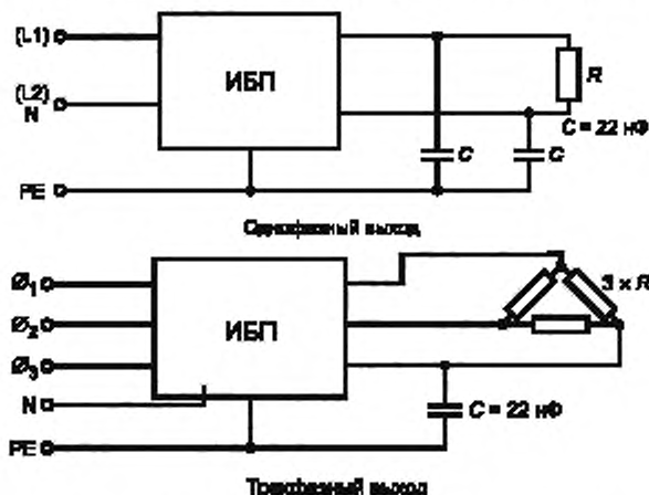
Рисунок L.1 — Схема подключения испытываемого ИБП
