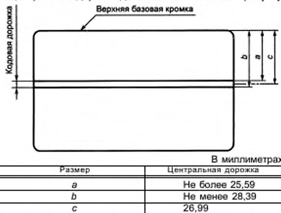
Рисунок 5 — Расположение центральной дорожки для формата TFC.1
