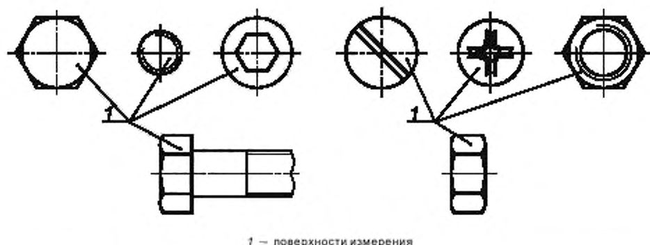
Рисунок 1 — Поверхности измерения локальной толщины покрытия на крепежных изделиях
