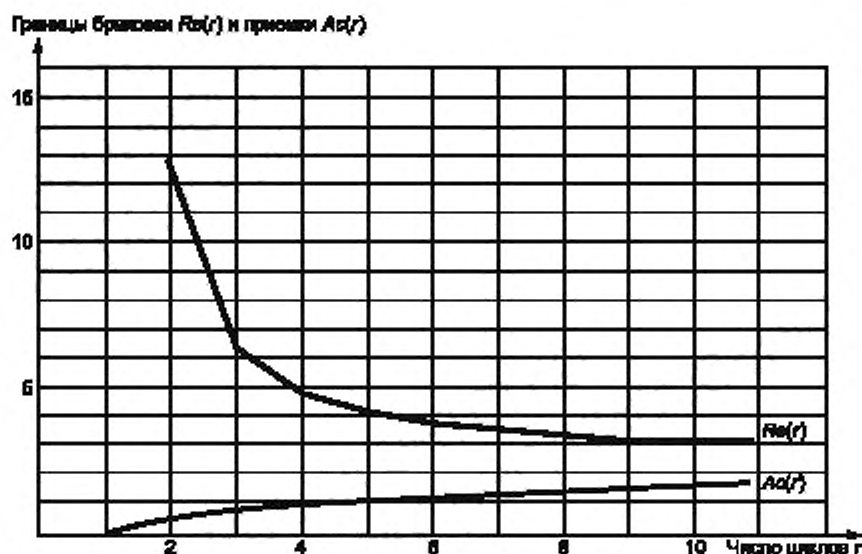
Рисунок 2 — Пример плана испытаний
