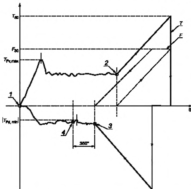
F — усилие предварительной затяжки; T — крутящий момент; \theta — угол поворота; 1 — точка, в которой впервые возникает стопорящий момент при закручивании и начинается измерение T_{Fv} ; 2 — точка лосадки, окончание измерений T_{Fv} ; 3 — отсутствие контакта с испытательной пластиной/шайбой, начало измерения T_{Fd} ; 4 — окончание измерения T_{Fd}
