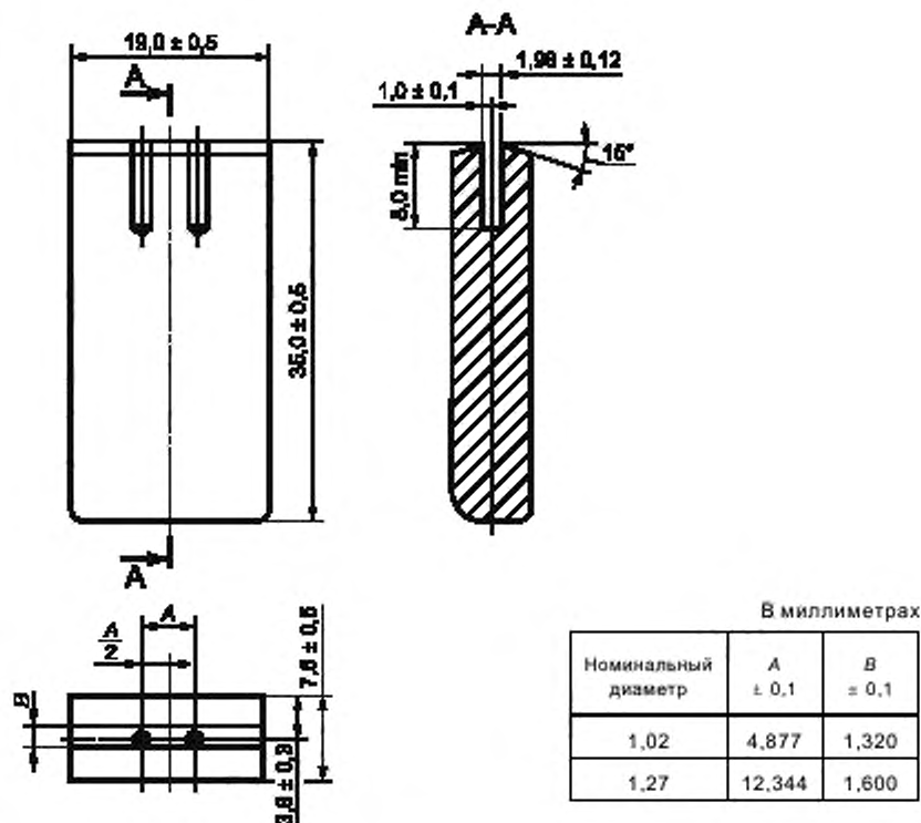
Рисунок 6 — Инструмент для испытания выводов на изгиб
