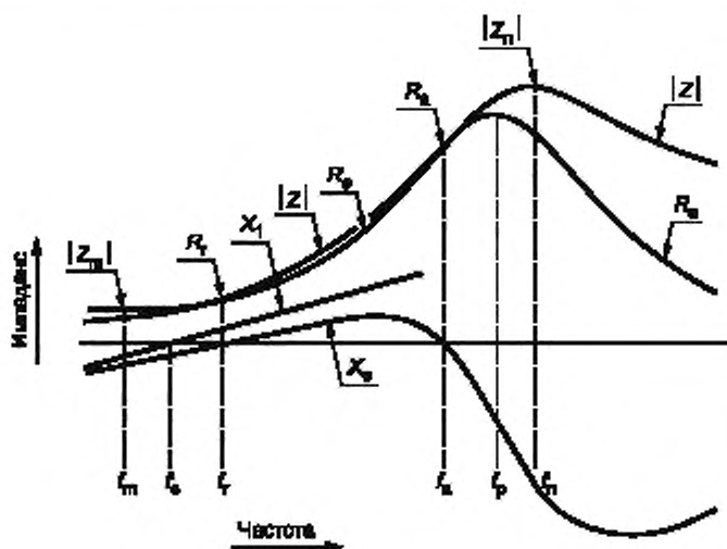
Рисунок 2 — Зависимость импеданса |Z| , активного сопротивления R_a , реактивного сопротивления X_a , сопротивления последовательной ветви X_1 пьезоэлектрического резонатора от частоты
