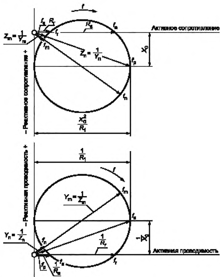
Рисунок 3 — Диаграмма импеданса и полной проводимости пьезоэлектрического резонатора
