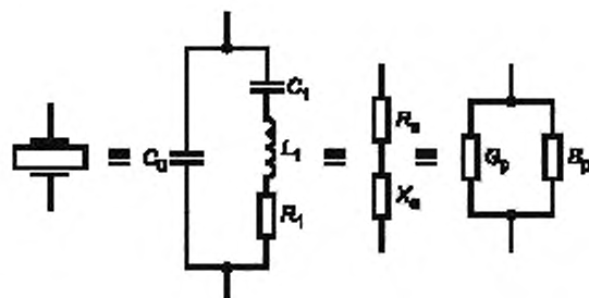
Рисунок 1 — Обозначения и эквивалентная электрическая схема пьезоэлектрического резонатора
