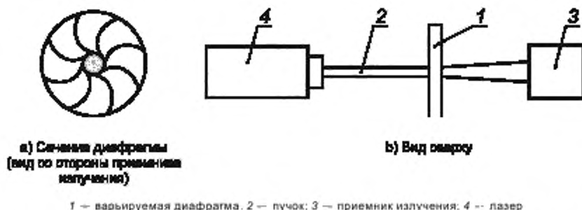
Рисунок 3 — Схема измерений ширины пучка по методике варьируемой диафрагмы
