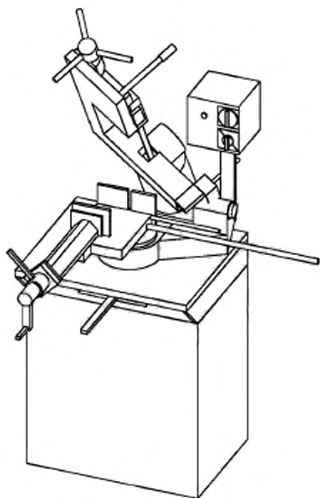
Рисунок С.2 — Горизонтальный ленточно-пильный станок с качающейся поворотной рамой
