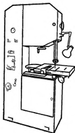
Рисунок С.4 — Вертикальный ленточно-пильный станок с неподвижной пильной рамой
