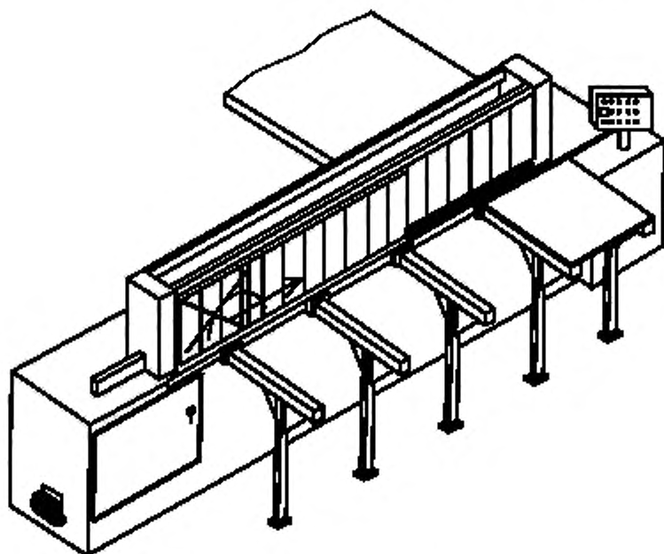
Рисунок С.10 — Круглопильный отрезной станок с продольно перемещающимся столом
