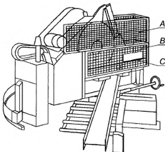
Рисунок D.4 — Ограждения на круглопильных отрезных станках с автоматическим соединенным шарниром, перемещаемым самозакрывающимся ограждением с противоударным смотровым окном, смежное с неподвижным ограждением, обеспечивающим закрытие дискового отрезного инструмента и рабочей зоны, а также самозакрывающиеся и неподвижные ограждения, закрывающие дополнительно разрезаемый материал, механизмы загрузки/разгрузки и подачи
