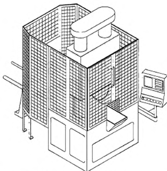
Рисунок D.6a — Ограждение на крупном круглопильном отрезном станке — полуавтомате вертикального типа
