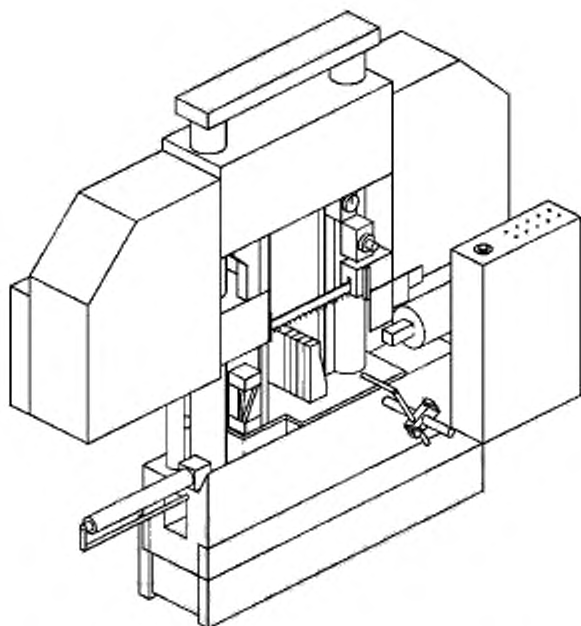
Рисунок С.3 — Горизонтальный ленточно-пильный станок колонного типа
