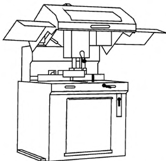
Рисунок С.9 — Круглопильный отрезной станок с подачей снизу вверх
