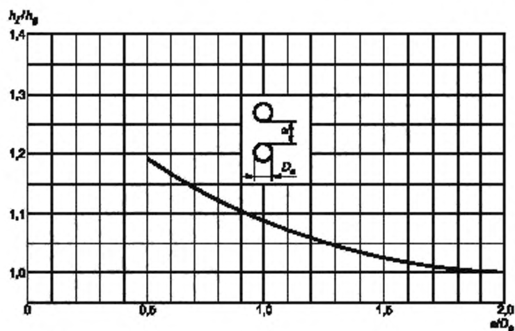
Рисунок 3 — Значения h_2/h_g для двух кабелей, расположенных в вертикальной плоскости
