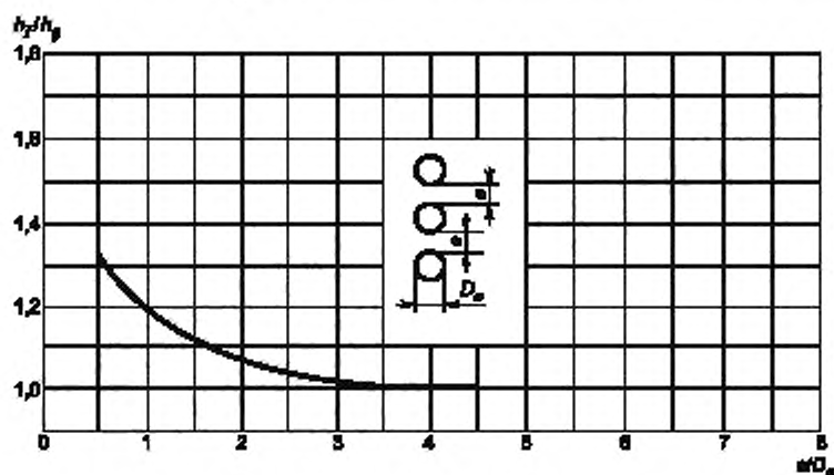
Рисунок 4 — Значения h_2/h_g для трех кабелей, расположенных в вертикальной плоскости
