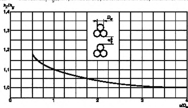
Рисунок 5 — Значения h_2/h_g для двух групп из трех кабелей, расположенных треугольником, в вертикальной плоскости
