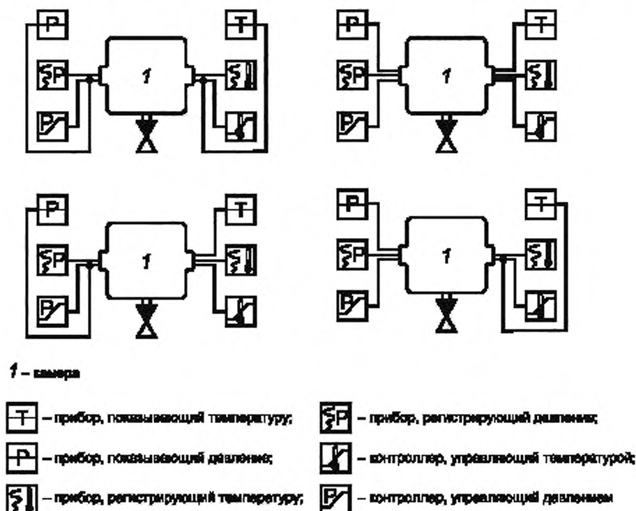
Рисунок 3 — Схемы организации подключения датчиков температуры и давления
