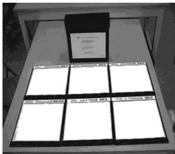
Рисунок 2 — Трехмерные эталоны гладкости
