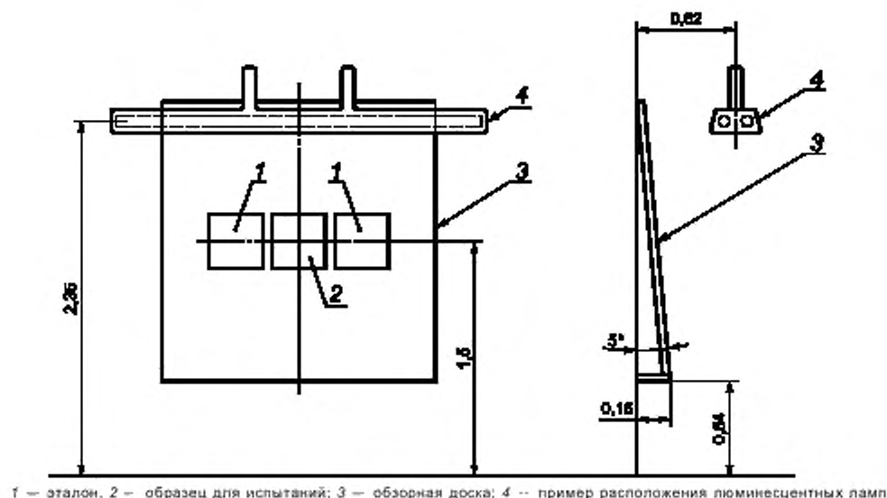
Рисунок 1 — Осветительное оборудование для просмотра образцов для испытаний
