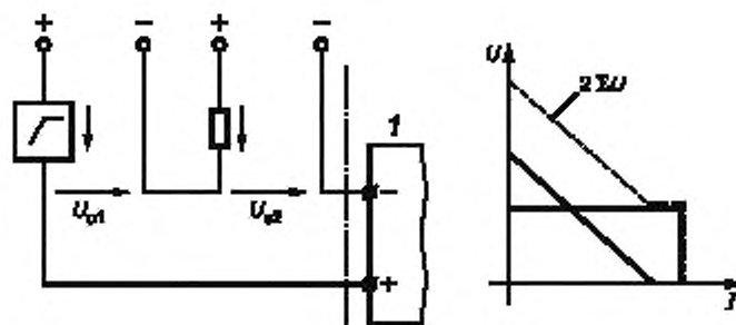
а — Последовательное подключение со сложением значений напряжения
