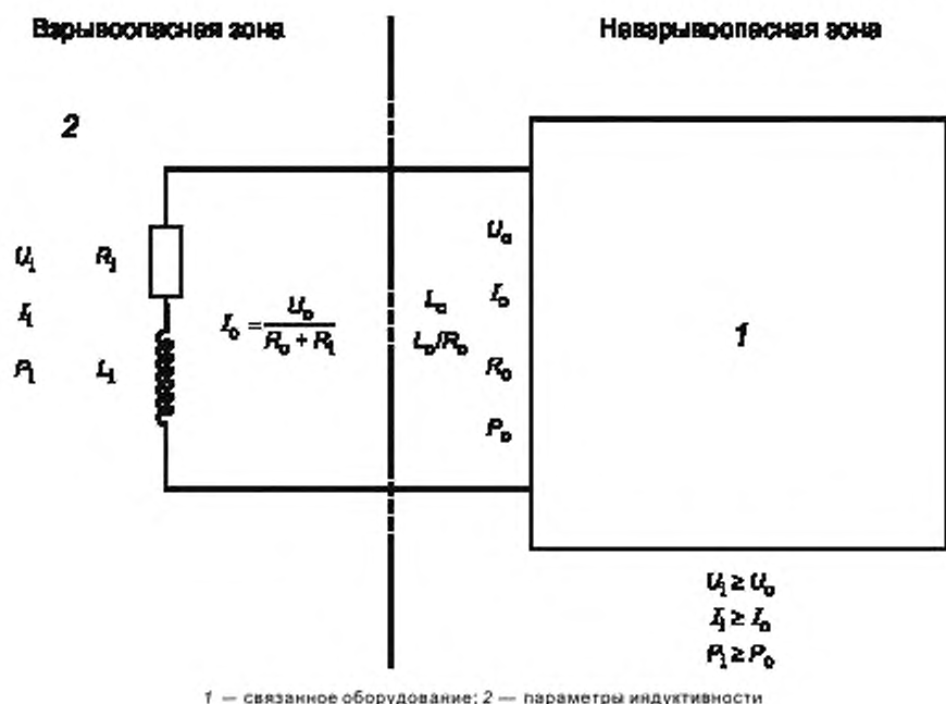
Рисунок D.1 — Типичная индуктивная цепь
