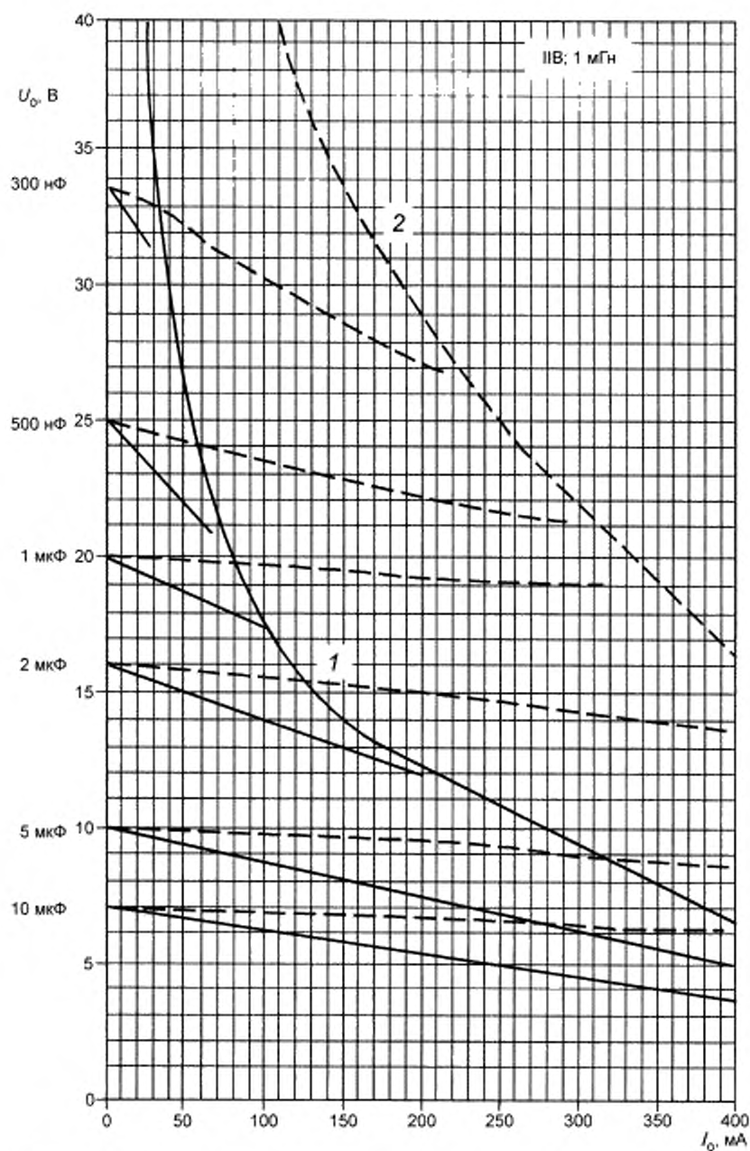
Рисунок С.8с — Диаграмма для значения 1 мГн
