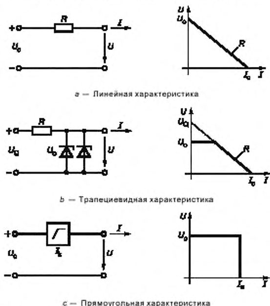
Рисунок С.1 — Характеристики эквивалентных цепей и выходов резистивных цепей
