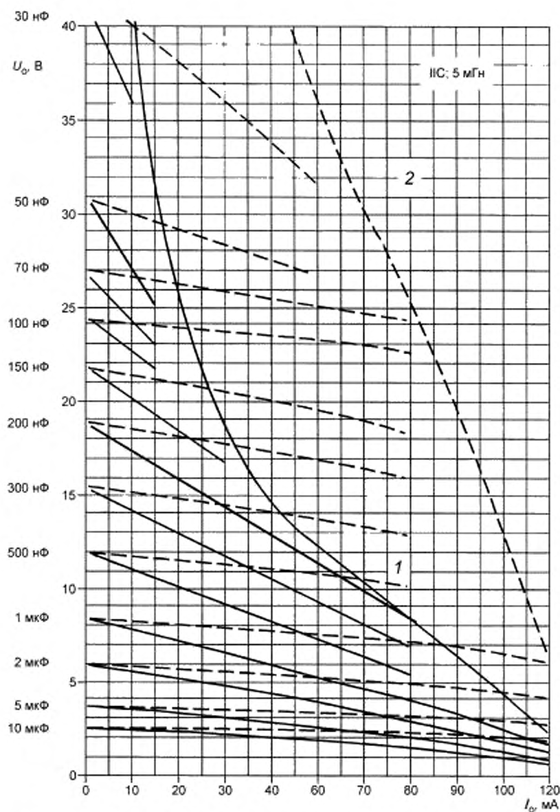
Рисунок С.7е — Диаграмма для значения 5 мГн
