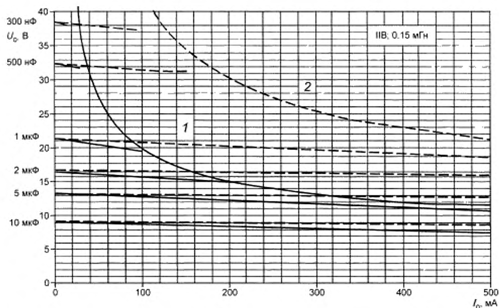
Рисунок С.8а — Диаграмма для значения 0,15 мГн (продолжение)
