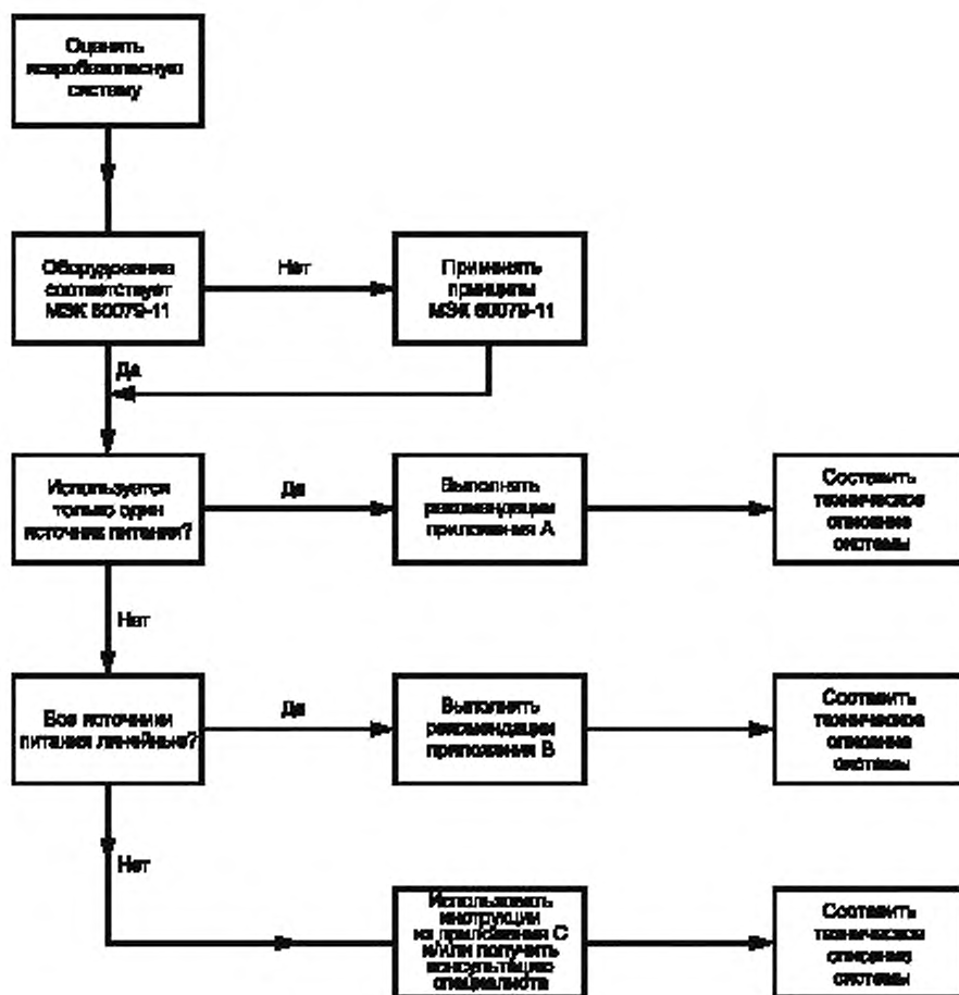
Рисунок 1 — Схема оценки системы
