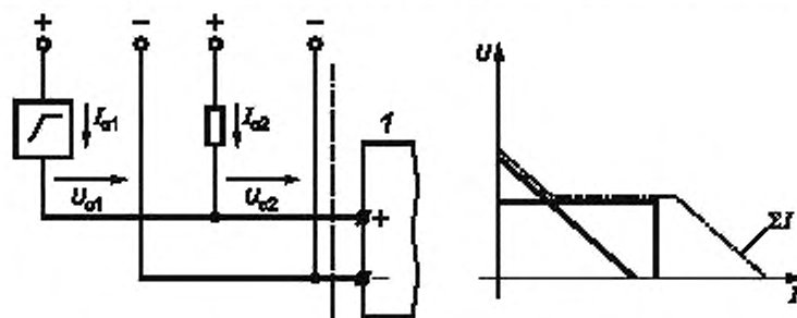
c — Параллельное подключение со сложением значений тока
