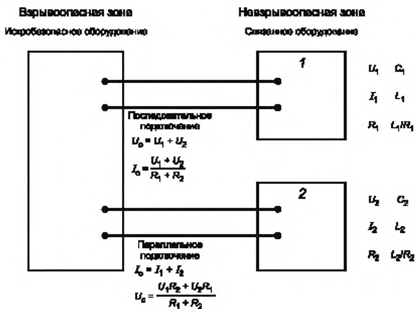
Рисунок В.3 — Источники питания, подключенные произвольно
