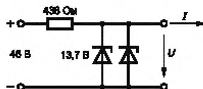
б — эквивалентная цепь
