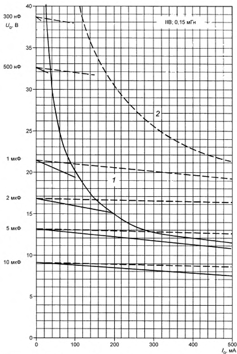
Рисунок С.8а — Диаграмма для значения 0,15 мГн
