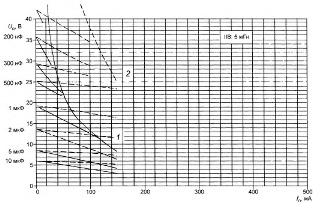
Рисунок С.8е — Диаграмма для значения 5 мГн (продолжение)
