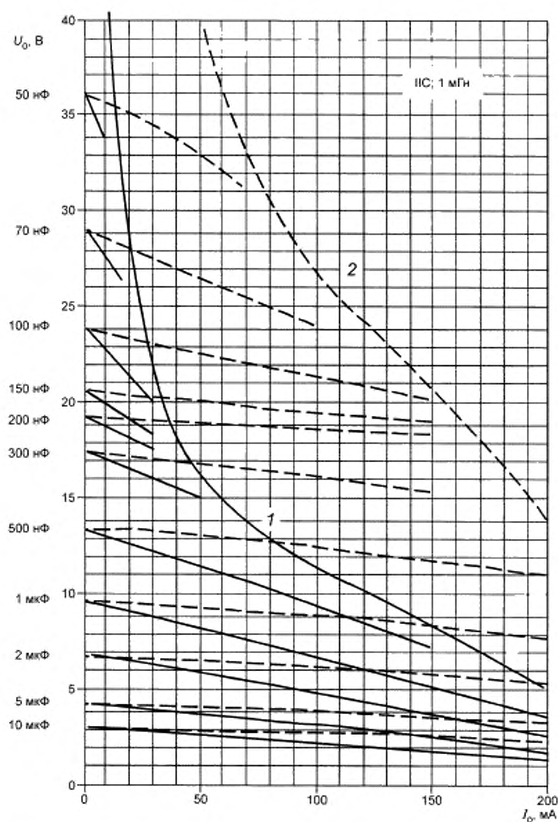
С.7с — Диаграмма для значения 1 мГн
