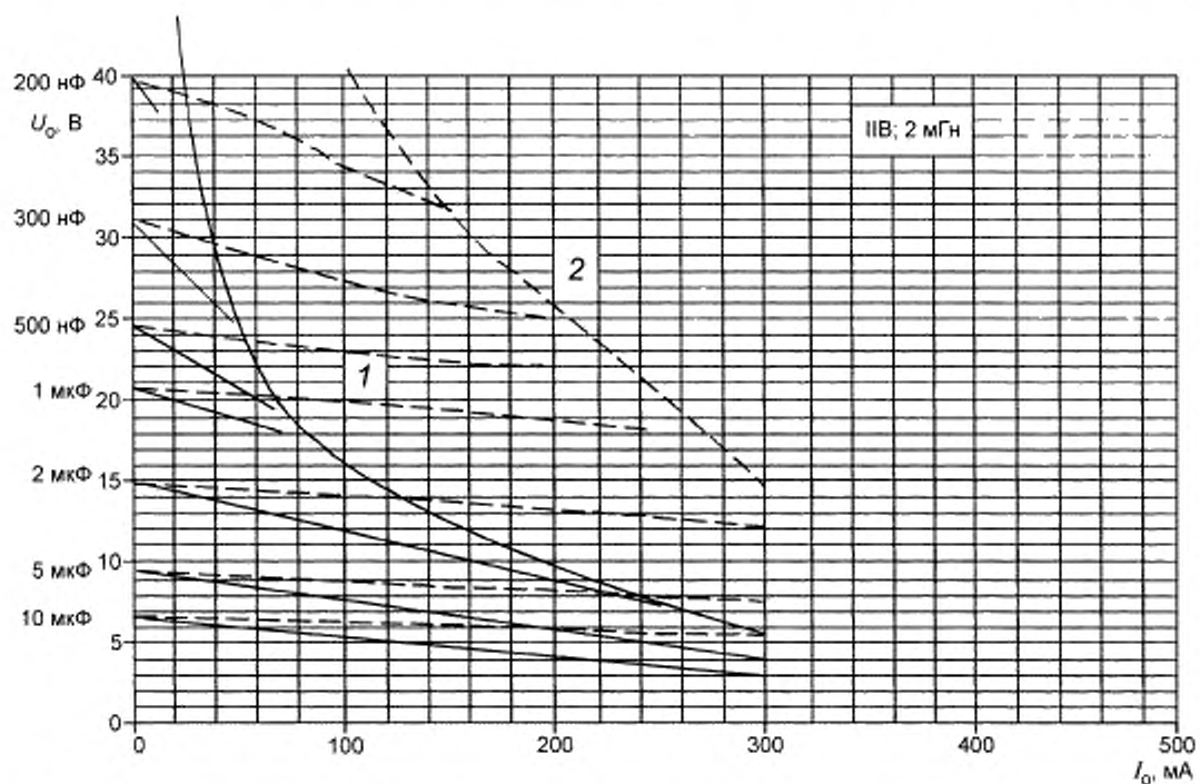
Рисунок С.8d — Диаграмма для значения 2 мГн (продолжение)
