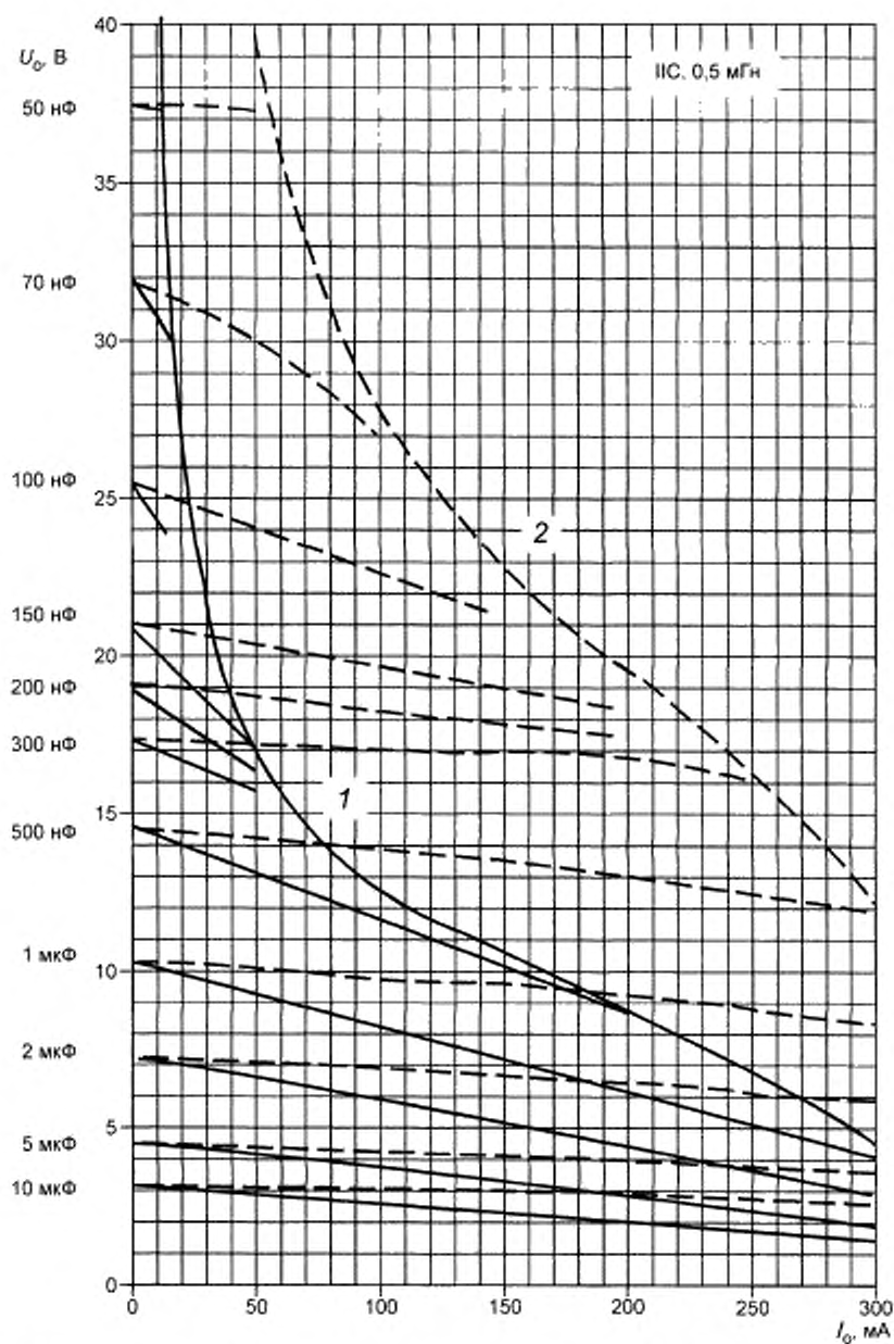
С.7b — Диаграмма для значения 0,5 мГн
