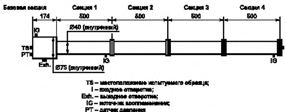
Рисунок 21 — Установка для испытаний дыхательных и дренажных устройств
