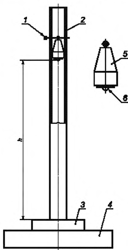
Рисунок С.1 — Пример установки для испытаний на ударостойкость
