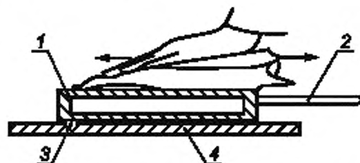
1 — поверхность А; 2 — тефлоновая ручка; 3 — поверхность В; 4 — фторопласт
