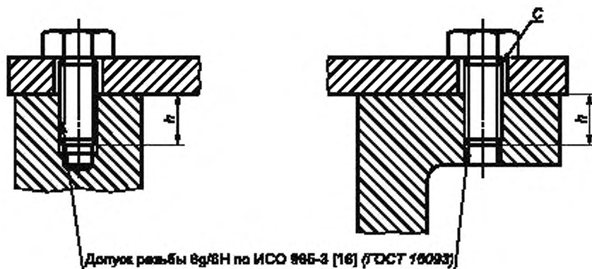
Рисунок 1 — Допуски и зазор для резьбовых крепежных деталей
