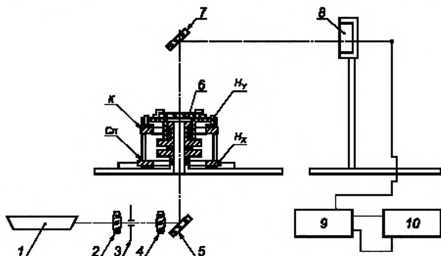
1 — лазер; 2, 4 — линзы; 3 — диафрагма; 5, 7 — плоское зеркало; 6 — испытуемое очковое стекло; 8 — фотоприемник; 9 — предварительный усилитель; 10 — двухкоординатный самописец; Сл — спираль; H_x , H_y — направляющие по осям x и y ; К — каретка
