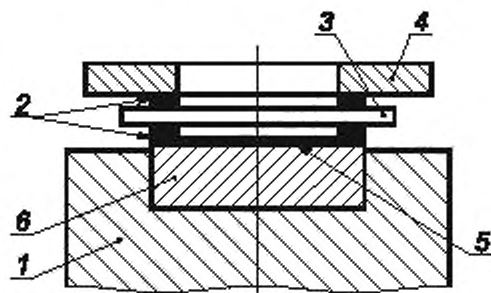
1 — станина; 2 — силиконовое опорное кольцо; 3 — испытуемое очковое стекло; 4 — нагрузочное кольцо; 5 — копирующая бумага, наложенная на белую бумагу; 6 — оправка под очковое стекло
