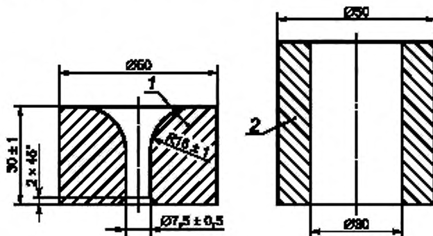
1 — воронка; 2 — цилиндр
