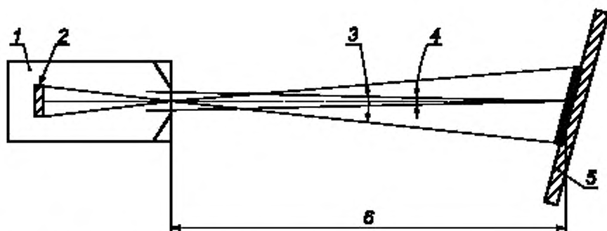
1 — фотометр; 2 — фотоэлектрический элемент; 3 — поле зрения: угловой размер рассматриваемого объекта, формируемый на приемнике; 4 — приемный конус: угол, формируемый входным лучом прибора на рабочем расстоянии; 5 — образец; 6 — рабочее расстояние: расстояние между передней линзой фотометра и объектом, на который сфокусирован фотометр
