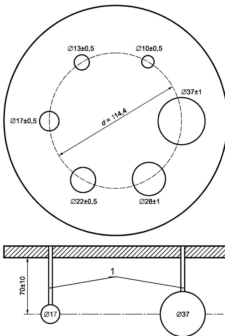
Рисунок 3 — Фантом руки
