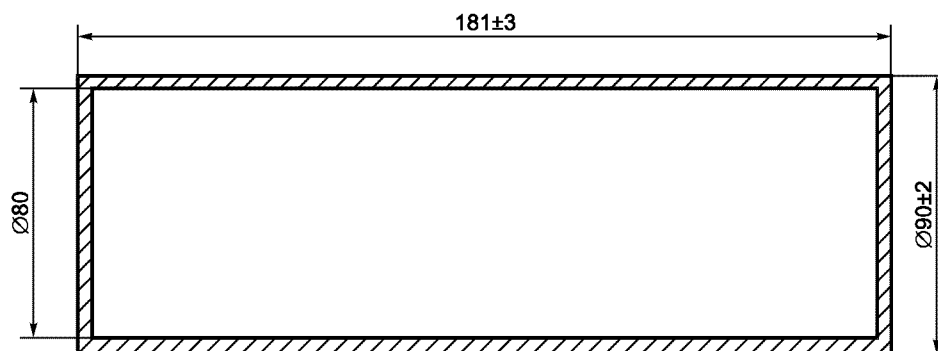
Рисунок 3 — Фантом руки
