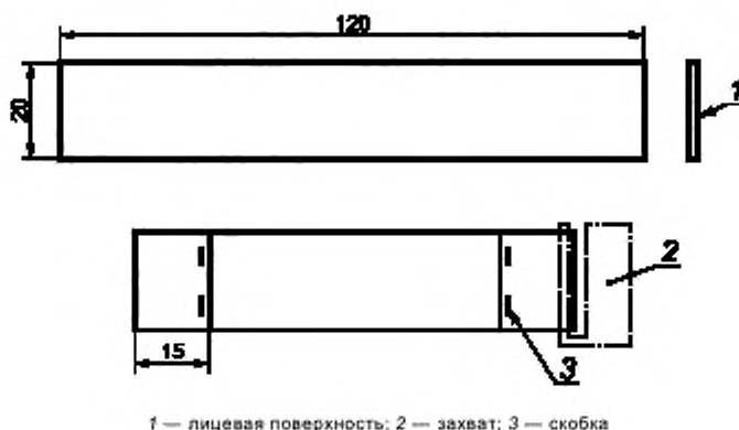
Рисунок 6 — Испытуемый образец
