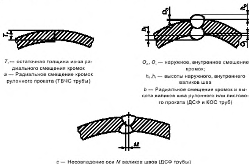
Рисунок 2 — Возможные отклонения размеров сварных швов
