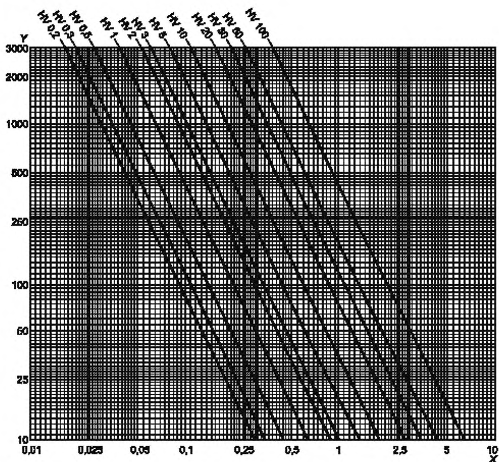
Рисунок А.1 — Минимальная толщина испытуемых образцов в зависимости от испытательной нагрузки и твердости (для шкал от HV 0,2 до HV 100)
