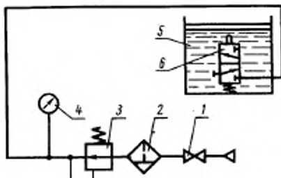
1—вентиль; 2—фильтр-высушитель; 3—регулятор давления; 4—образцовый манометр; 5—испытываемый пневмораспределитель; 6—бачок с эмульсией
