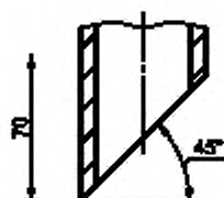
Рисунок А.6 — Штыцер и уплотнительное кольцо датчика температуры
