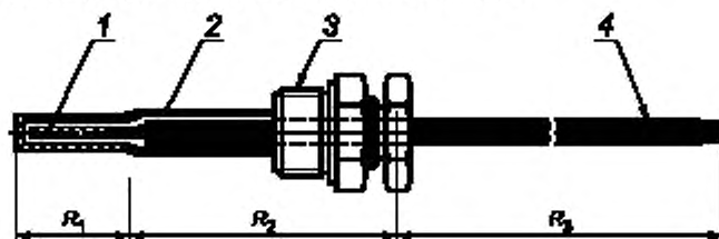
Рисунок 5 — Датчик температуры с постоянно присоединенным кабелем
