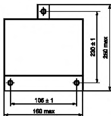
Рисунок 8 — Габаритные размеры, мм
