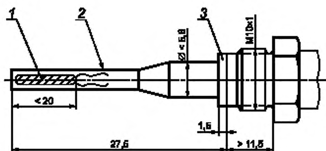
1 — термочувствительный элемент; 2 — защитный корпус; 3 — уплотнительное кольцо
