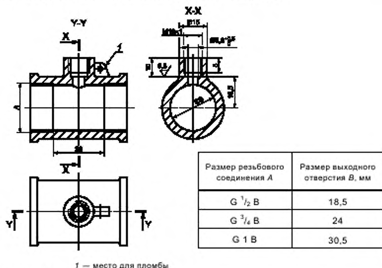
Рисунок А.6 — Штыцер и уплотнительное кольцо датчика температуры
