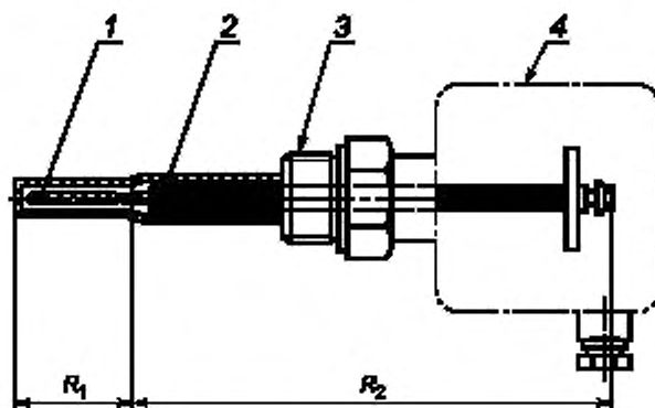
Рисунок 6 — Датчик температуры с соединительной головкой
