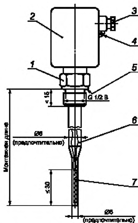
1 — зажимная гайка; 2 — головка (типичная); 3 — вход для кабеля сигнала; 4 — место для опломбирования; 5 — поверхность уплотнения; 6 — защитный корпус датчика температуры; 7 — термочувствительный элемент
