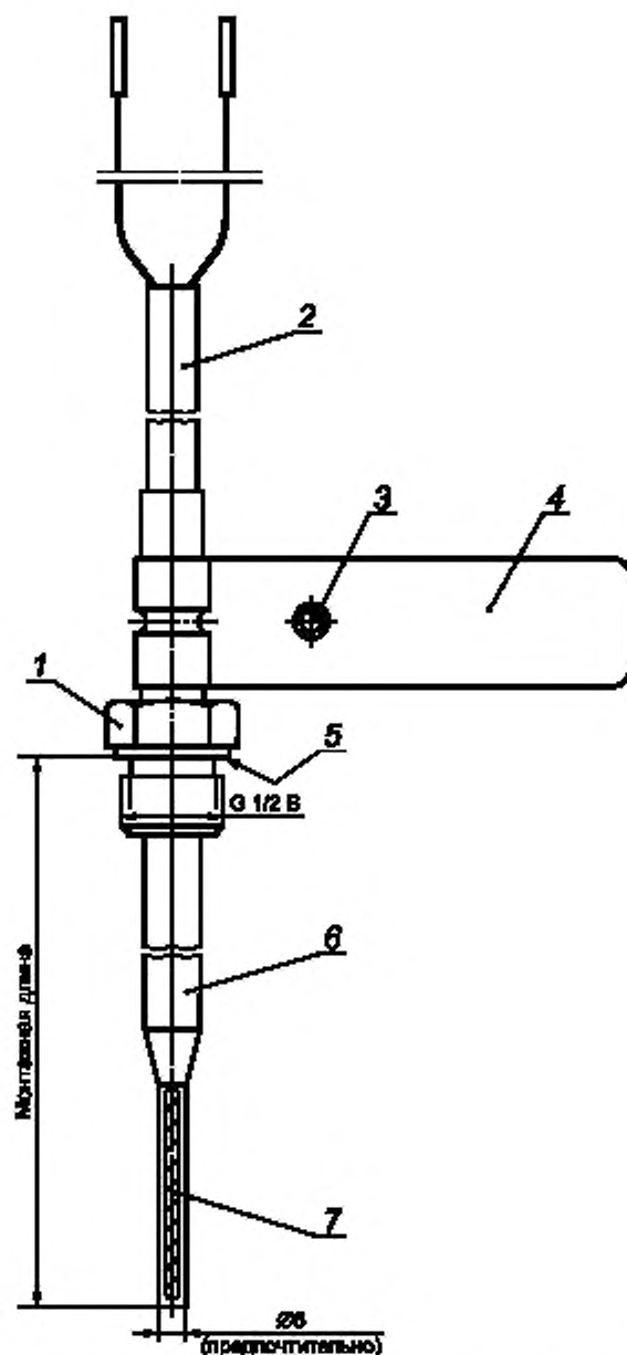
1 — зажимная гайка; 2 — соединительный кабель; 3 — место для опломбирования (пример); 4 — идентификационная пластина (пример); 5 — поверхность уплотнения; 6 — защитный корпус датчика температуры; 7 — термочувствительный элемент
