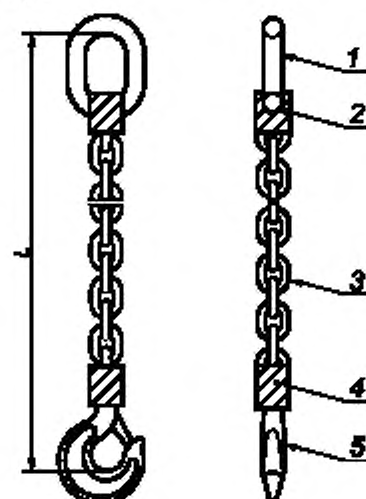
а) Смонтированная стропальная цепь из одного жгута
