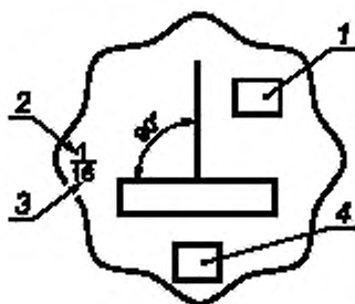
Рисунок D.1 — Ярлык для маркировки стропальных цепей из одного жгута
