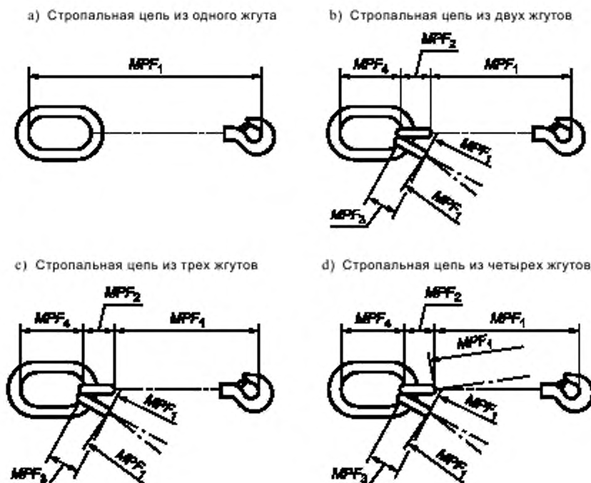
Рисунок 6 — Испытательные участки стропальных цепей
