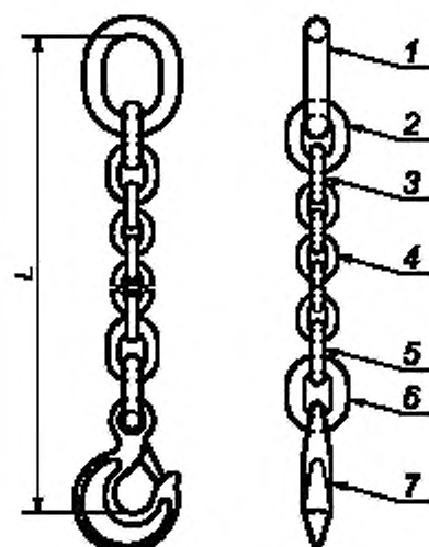
б) Сварная стропальная цепь из одного жгута
