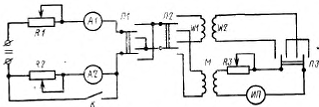
R_1, R_2 — регулировочные устройства; A_1, A_2 — амперметры; П_1, П_2, П_3 — двухполюсные переключатели; K — ключ; W_1 — намагничивающая обмотка образца или намагничивающего устройства; M — образцовая катушка взаимной индуктивности; R_3 — магазин сопротивлений; ИП — баллистический гальванометр или веберметр; W_2 — измерительная обмотка образца или измерительная катушка
