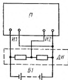
ДН — делитель напряжения Черт. 3
