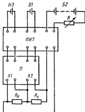
\Pi — потенциометр постоянного тока; \Pi NT — переключатель направления тока; R_0 — образцовая мера сопротивления; R_x — измеряемое сопротивление; R — декалибровочный матазан сопротивления; H3 — нормальный элемент; B_1 , B_2 — источники питания.
