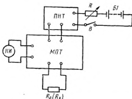
МПТ—мост постоянного тока; НИ—нулевой индикатор
