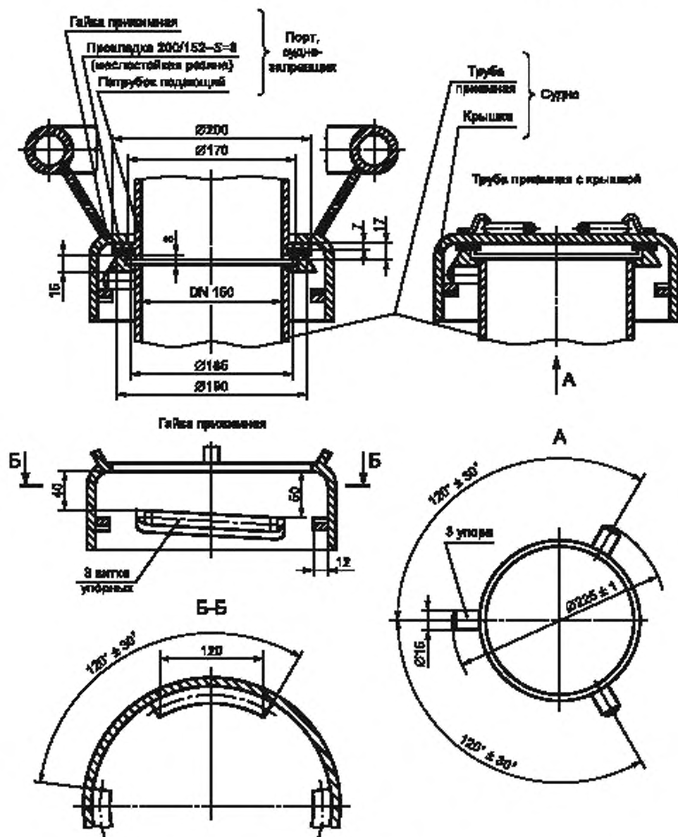
Рисунок 2 — Устройство для приема топлива номинальным диаметром 150 мм
