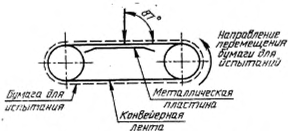
Рисунок 1 — Схема испытательного устройства
