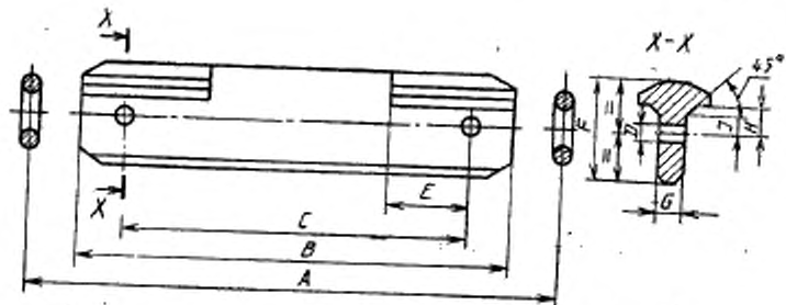
Рисунок 1 — Размеры Т-образных скребков
