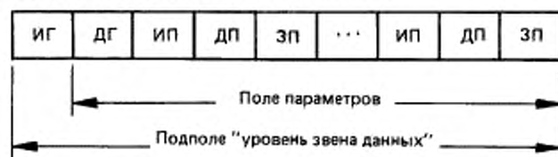
Рисунок 3 — Типичный формат подполя «уровень звена данных»
