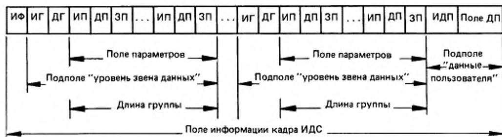
Рисунок 5 — Структура поля информации кадра ИДС
