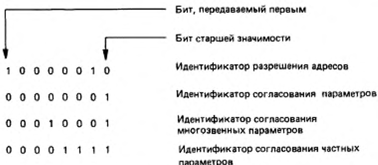
Рисунок 7 — Кодирование подполя «уровень звена данных»
