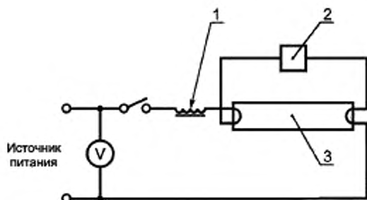
Рисунок A.1 — Схема испытания на зажигание со стартером
