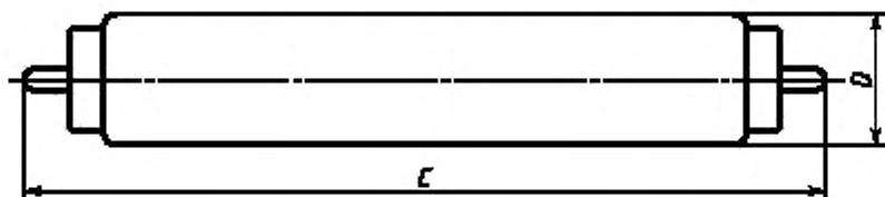
Цоколь Fa6 по МЭК 60061-1
