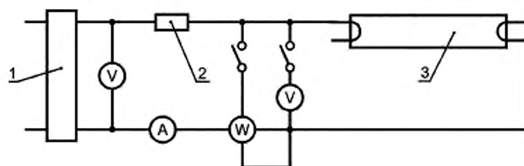
1 — ВЧ генератор; 2 — образцовый ПРА; 3 — лампа
