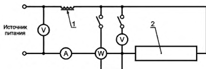
1 — образцовый ПРА; 2 — лампа
