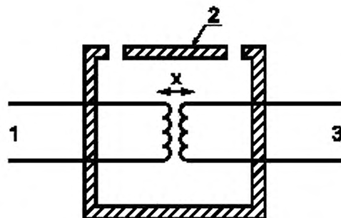
1 — опасная цепь 1; 2 — доступная часть, не связанная с зажимом защитного заземления; 3 — опасная цепь 2
