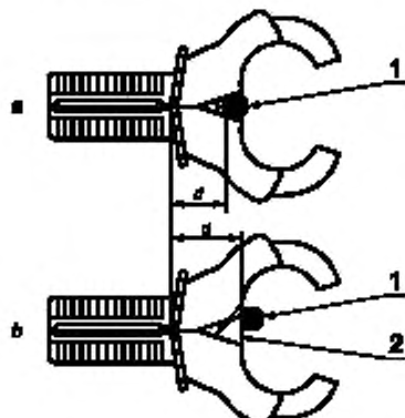
Рисунок 103 — Минимальные зазоры между защитным ограждением и проводником при разомкнутых амперометрических клещах
