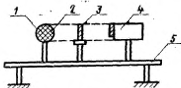
1 — изотопный источник быстрых нейтронов; 2 — шаровой замедлитель; 3 — кадмевый экран; 4 — блок детектирования; 5 — градуировочная линейка
