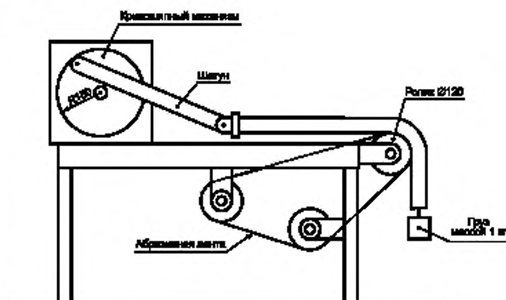
Рисунок 101 — Устройство для испытаний токоведущих шлангов на устойчивость к истиранию
