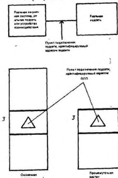
Рисунок 1 — Адрес подсети
