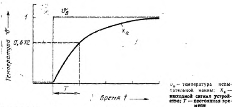
Рисунок BB1 — Определение постоянной времени методом быстрого изменения температуры
