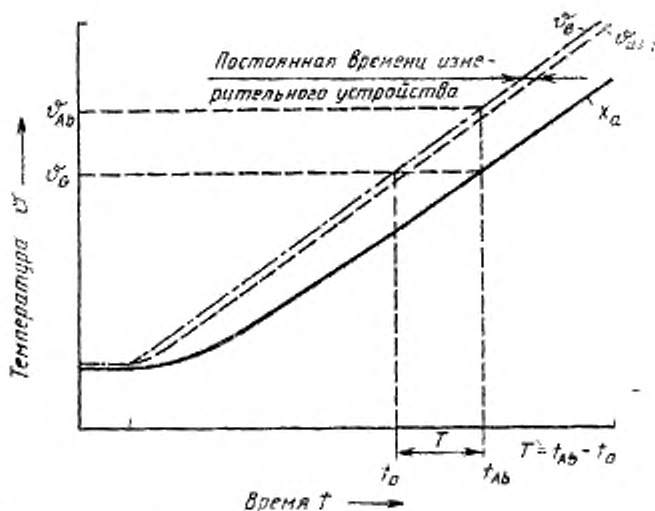
Рисунок BB1 — Определение постоянной времени методом быстрого изменения температуры
