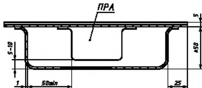
Рисунок 6 — Испытательный корпус для тепловых испытаний ПРА
