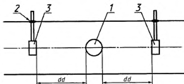
1 — нормальное расположение температурного датчика системы увлажнения; 2 — заглушка; 3 — стандартный датчик температуры
