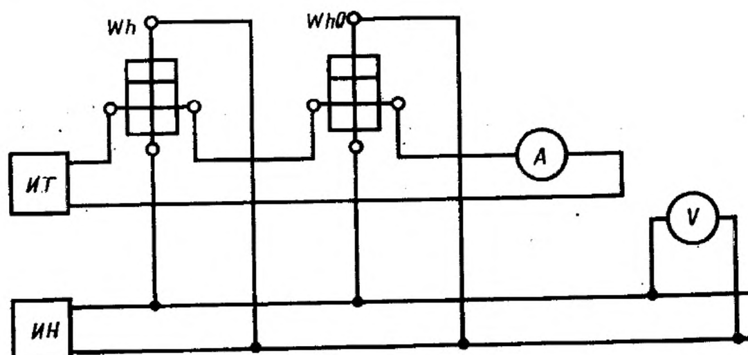
Wh —поверяемый счетчик; Wh_0 —образцовый счетчик; ИТ—источник постоянного тока; ИН—источник постоянного напряжения; А—образцовый амперметр; V—образцовый вольтметр
